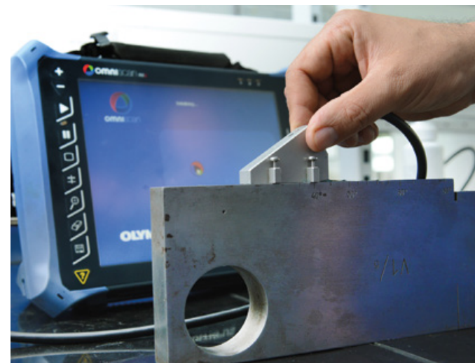
Ultraschall-Phased-Array-Prüfung an einem Vergleichskörper
